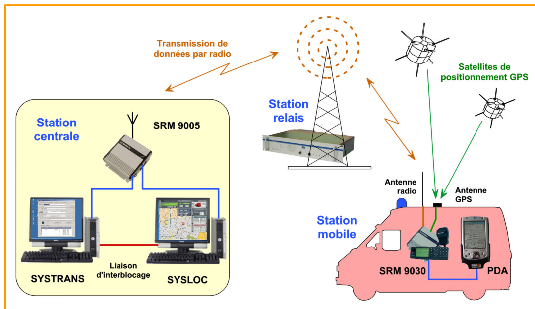
Configuration des deux systèmes SYSTRANS et SYSLOC en cohabitation
